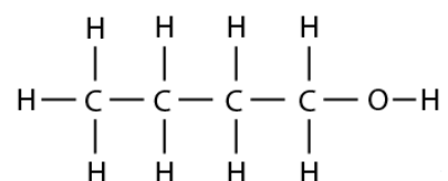
Butan-1-ol
